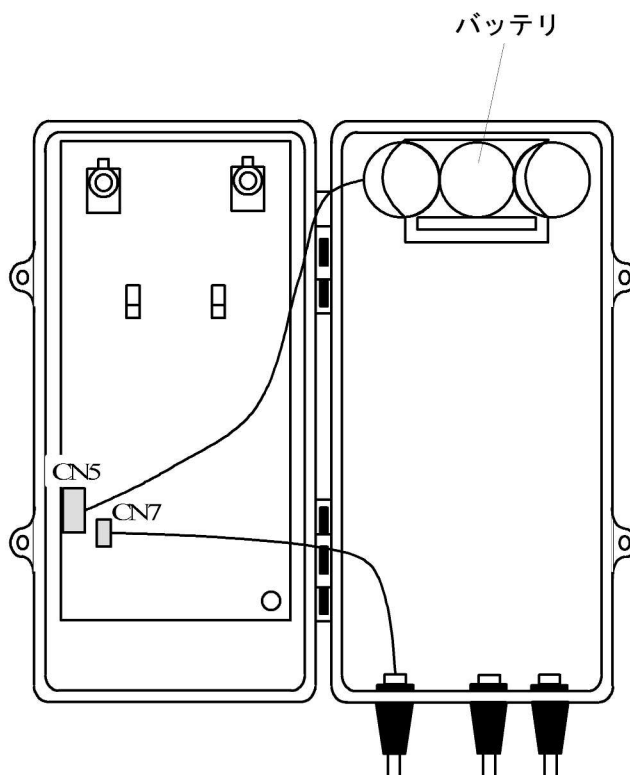
時計駆動器内部コネクタ配置図
